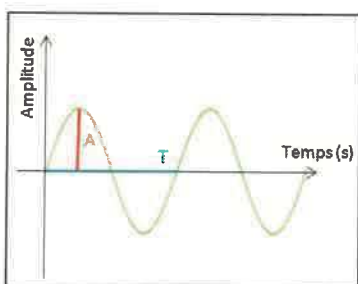
Figure 5 : représentation d'un son simple (son pur)
