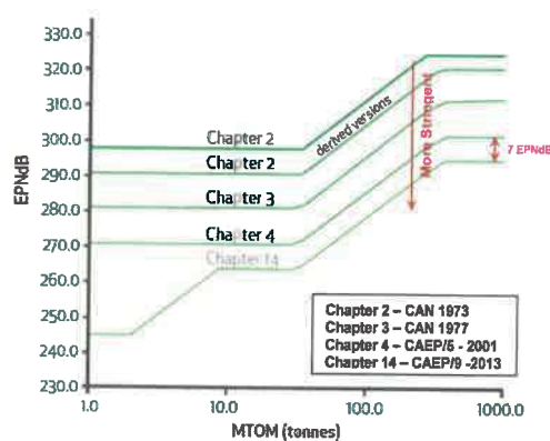
Figure 10 : niveau de bruit par chapitre OACI en fonction de la MTOW - Source : OACI
